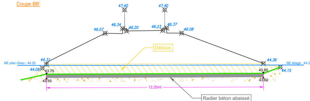
Vue de profil prise d'eau
