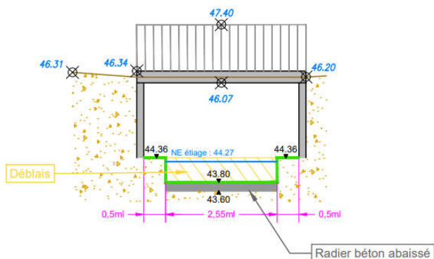
Vue de face prise d'eau
